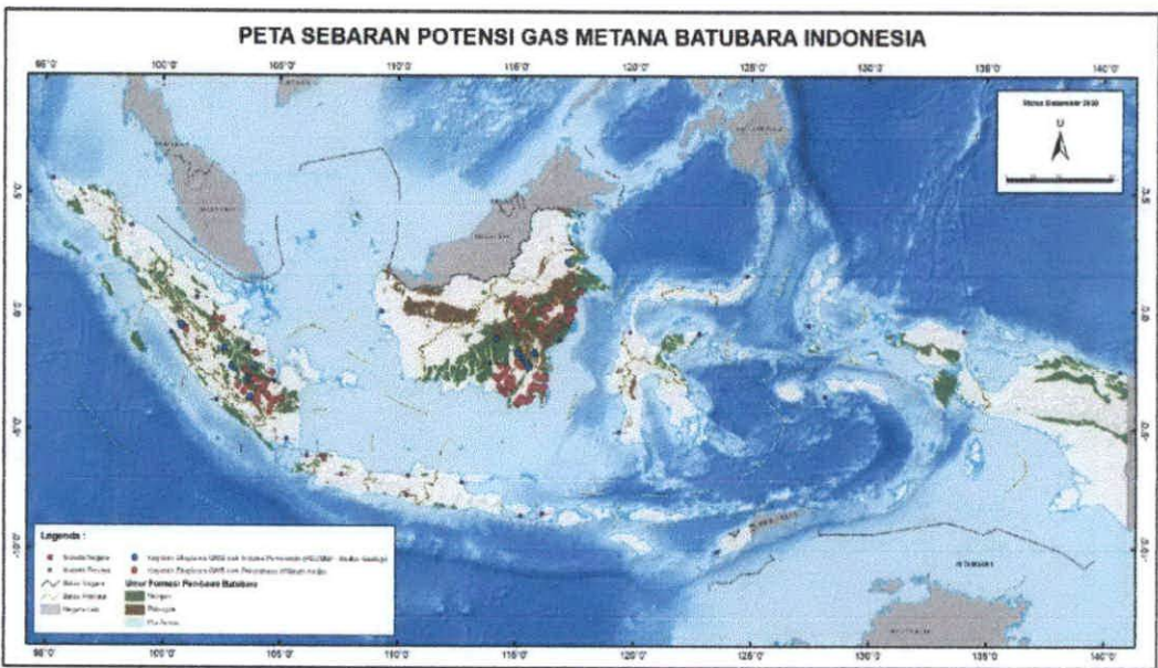
Gambar I.2.2 Peta Sebaran Potensi Gas Metana Batubara Indonesia
