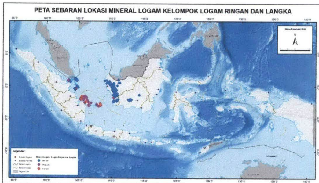
Gambar I.1.3 Peta Sebaran Lokasi Mineral Logam Kelompok Logam Ringan dan Langka
